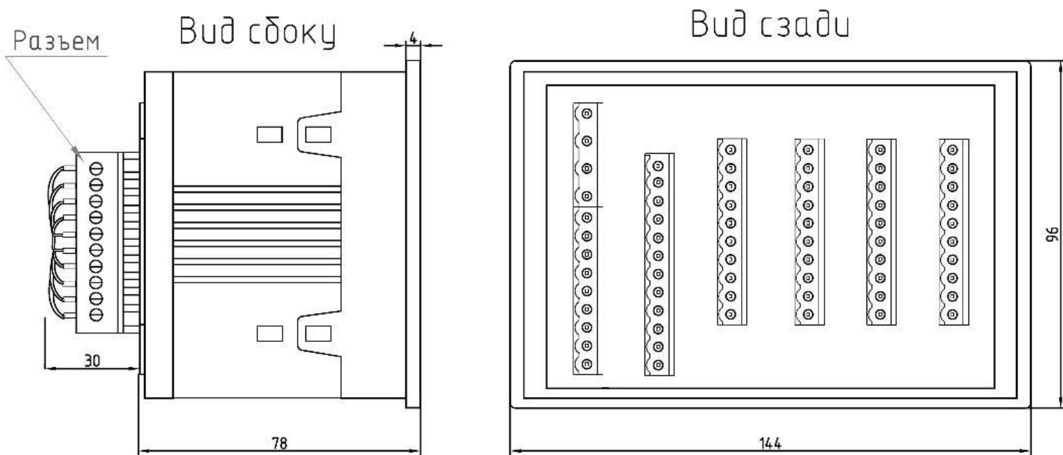
Рисунок 10. Размеры изделия, необходимые для его монтажа.
