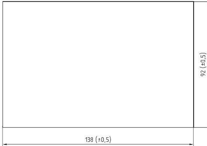
Рисунок 9. Требуемые размеры окна для установки контроллера.
